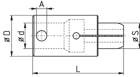
Spannhülse - collet
